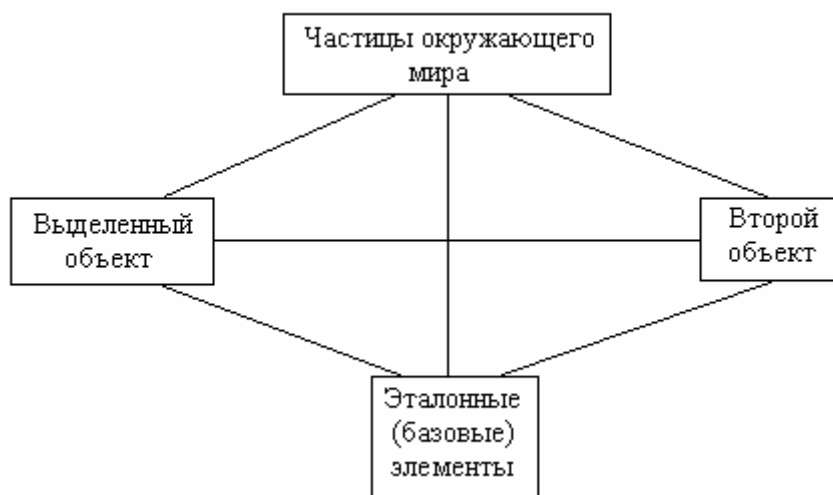
Рис. VI. 2. Четыре характерных подмножества элементов теории.
