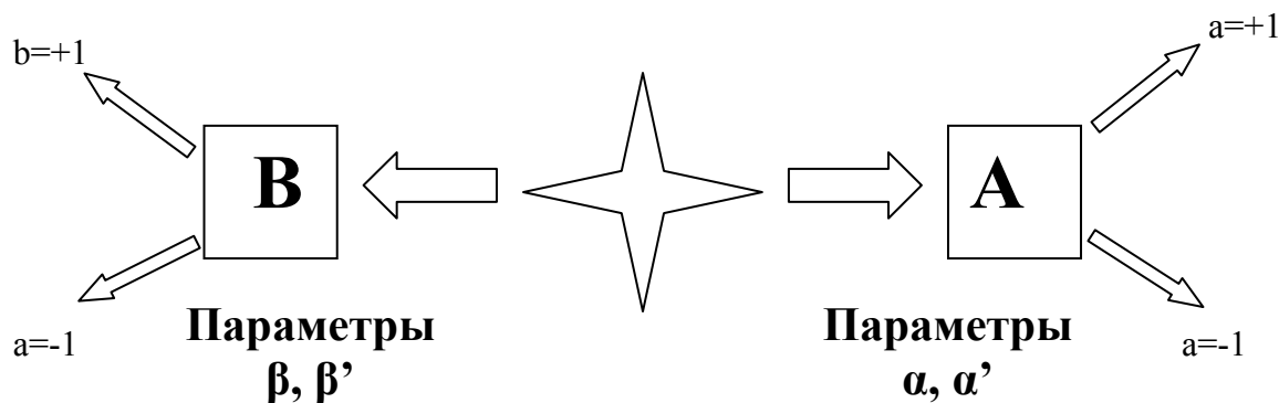
Рис. II.1 Эксперимент по проверке неравенства Белла.
