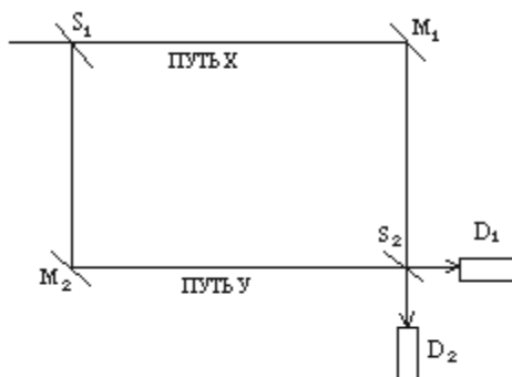
Рис III. 2. Нейтронный интерферометр.
