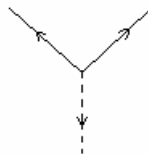
Рис. IV.1 Рождение виртуальной частицы.
