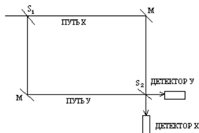
Рис. II.1 Схема эксперимента Уилера
