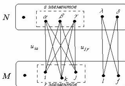
Рис. VI.1. Бинарная система отношений (структура) ранга (r,s).
