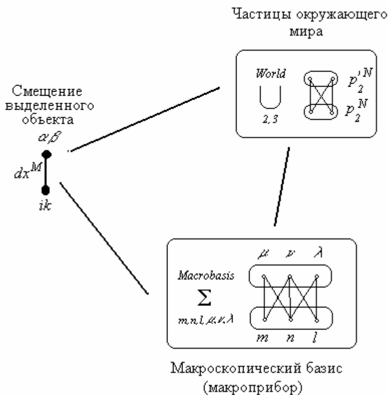
Рис.V. 3. Усреднение парного отношения выделенного объекта по ансамблю базисных элементов, составляющих макроприбор.
