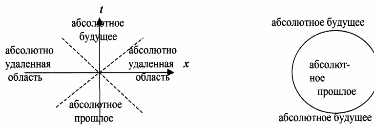
Рис.4. Области 4-мерного континуума в СТО (слева) и ТШРВ (справа).
