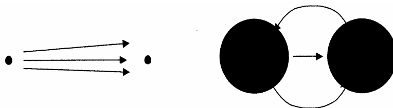
Рис.1. Слева – локально однородное поле тяготения, справа – поле, которое нельзя считать однородным даже локально.
