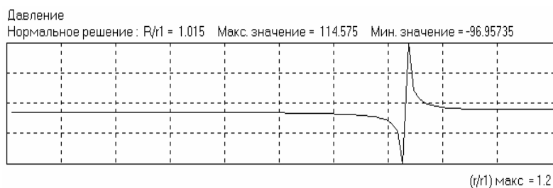
Рис.2. Характер изменения давления в непосредственной близости от пограничного коллапса. По оси ординат отложено безразмерное давление, по оси абсцисс – отношение расстояния r от центра шара к радиусу шара r_1 . В данном случае коллапс не наступает, поскольку отношение радиуса кривизны R больше радиуса шара r_1 .
