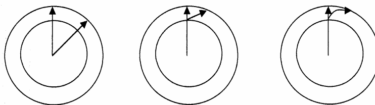
Рис.3. Эффект "перемещения" точек на поверхности гиперсферы для неподвижных в пространстве объектов (слева), движущихся по инерции (в центре) и ускоренно (справа).
